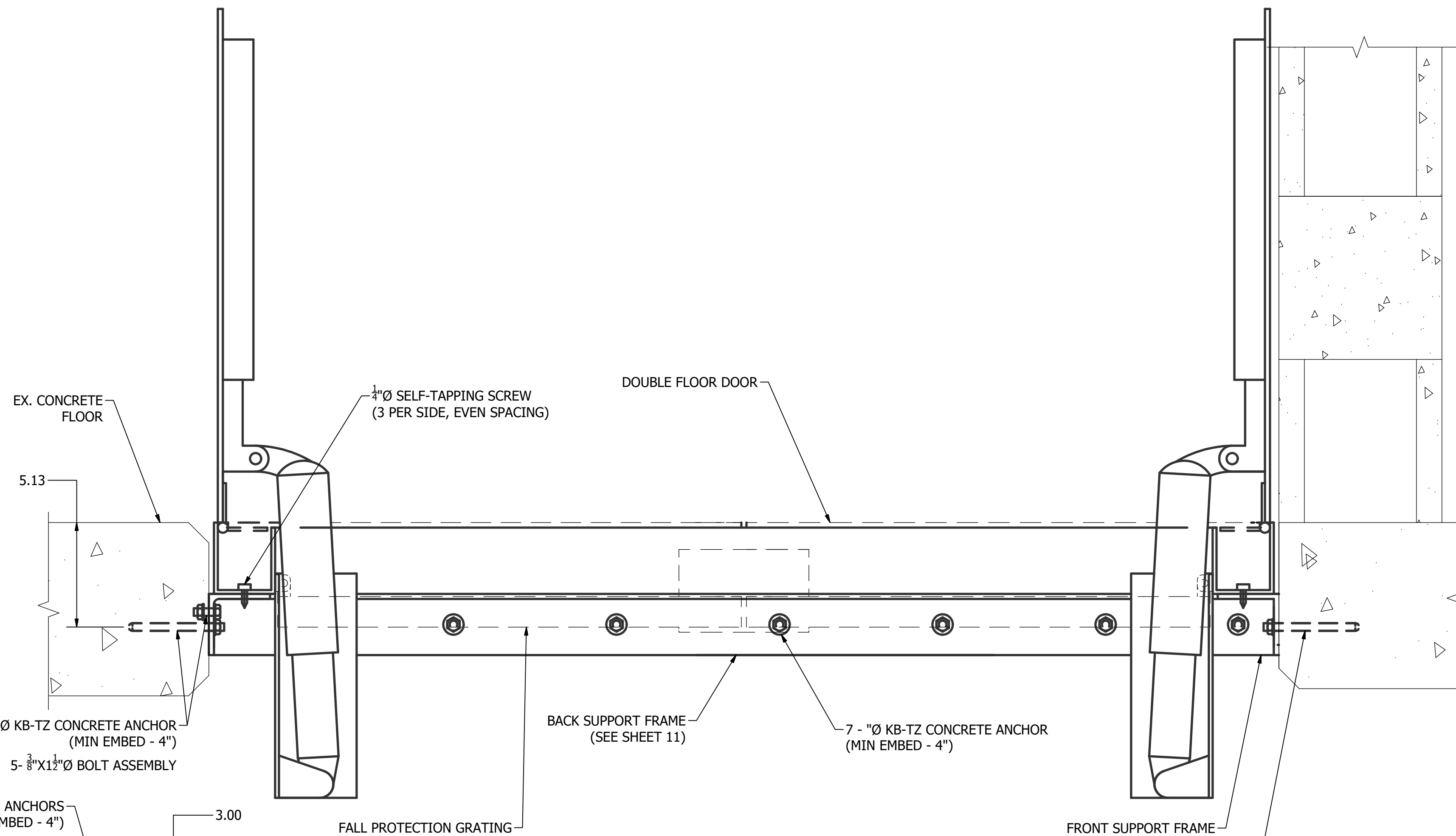
SECTION A-A
